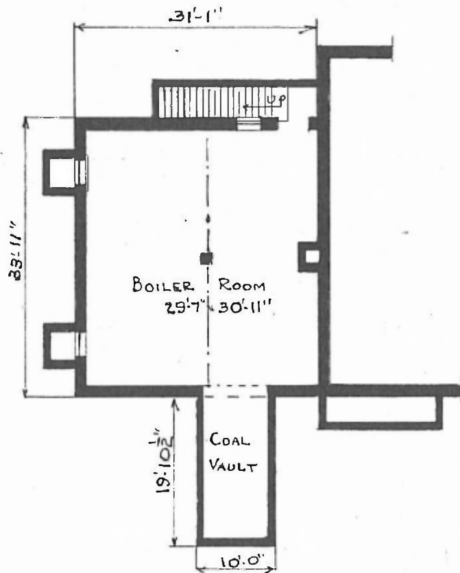
BOILER ROOM SCALE: \frac{1}{16}'' = 1'-0''
