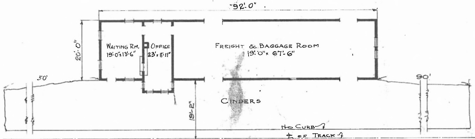
FLOOR PLAN SCALE: \frac{1}{16}'' = 1'-0''
