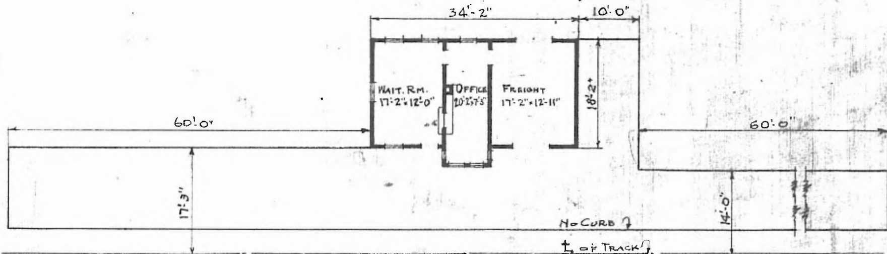
FLOOR PLAN SCALE: \frac{1}{16}'' = 1'-0''
