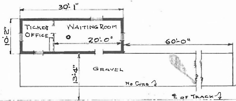
FLOOR PLAN SCALE: \frac{1}{16}'' = 1'-0''
