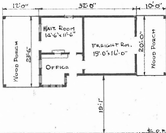
FLOOR PLAN SCALE: \frac{1}{16} = 1'-0''
