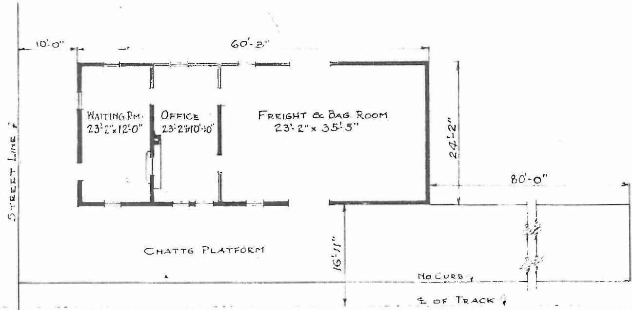
FLOOR PLAN SCALE: \frac{1}{16}'' = 1'-0''
